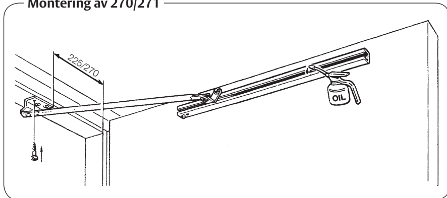
Montering av 270/271
