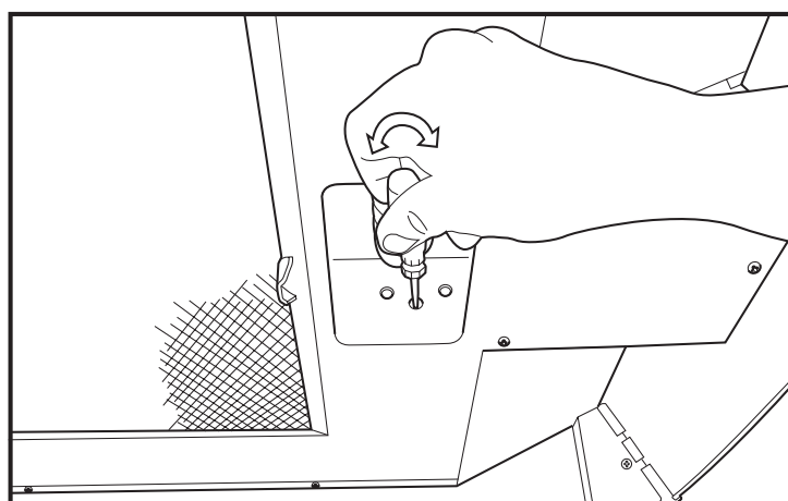
2. Använd en skruvmejsel för att ställa in tilluftstemperaturen efter ventilationsaggregatet. Denna är vid leverans inställd på 10° C.
