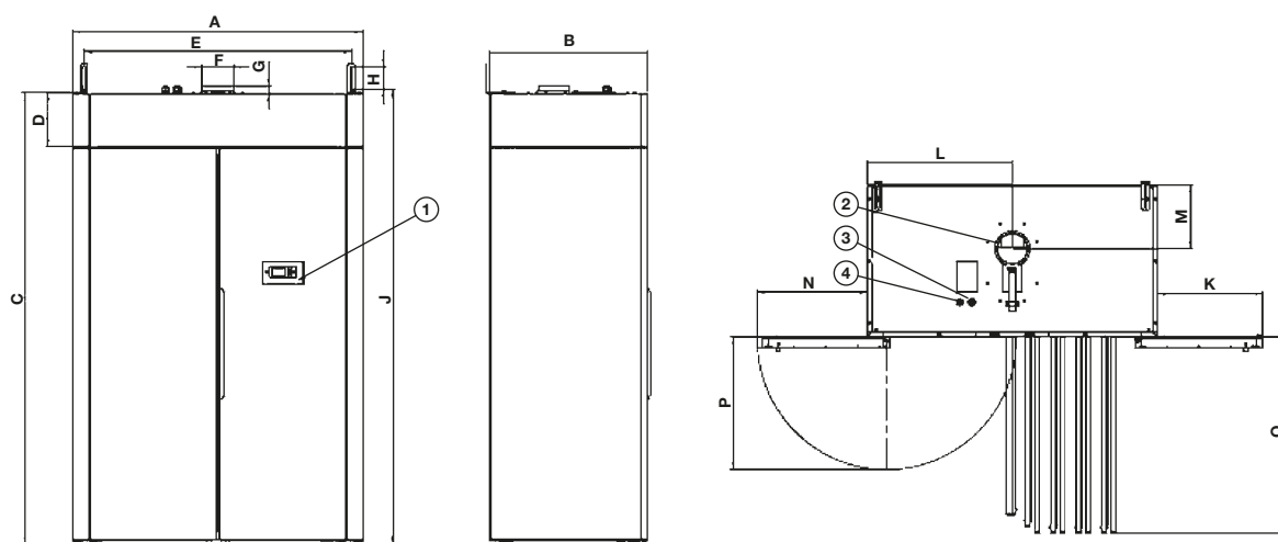
① Manöverpanel ② Frånluftsanslutning ③ Elanslutning nät ④ Elanslutning extern fläkt
