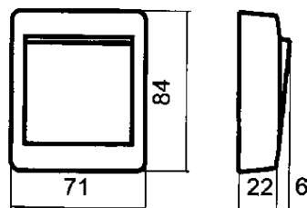
Måttritning
